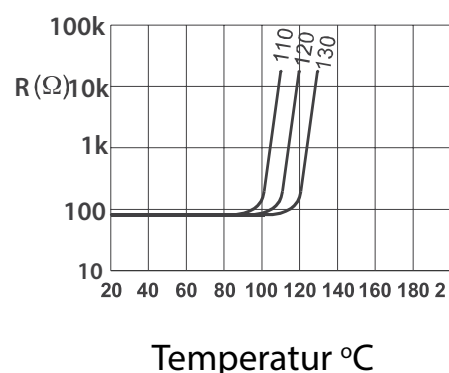
Typischer Widerstand von PTC im Vergleich zu * Temperatur-Kennlinien-Grafik
